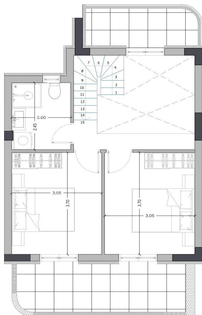
Α' ΟΡΟΦΟΣ
