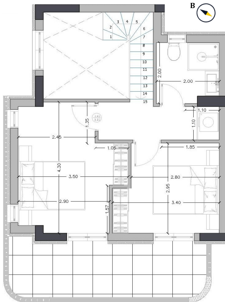
Α' ΟΡΟΦΟΣ
