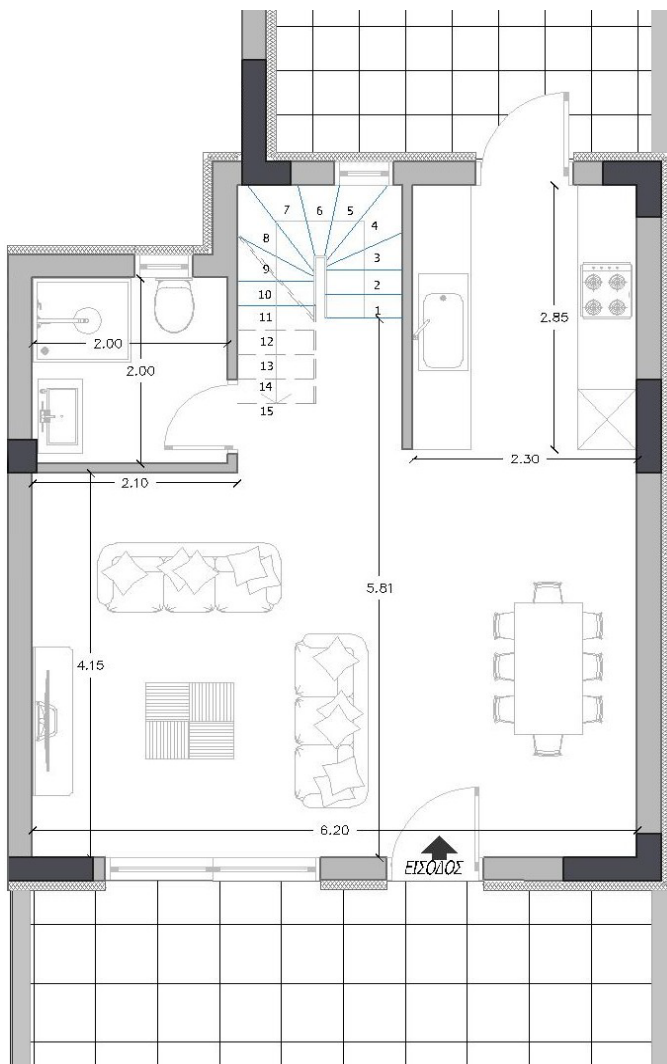
ΙΣΟΓΕΙΟ
