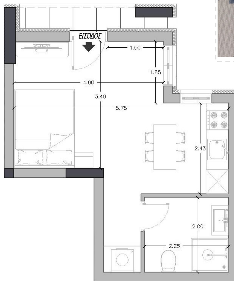
ΚΑΤΟΨΗ ΔΙΑΣΤΑΣΕΙΣ
