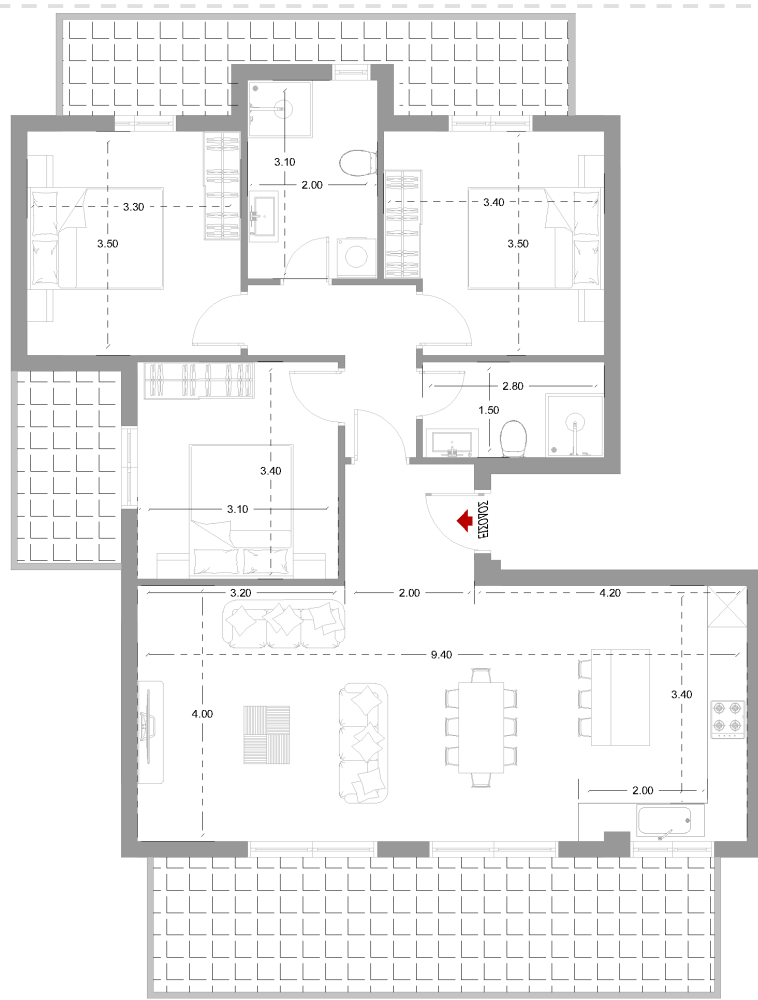
ΚΑΤΟΨΗ ΔΙΑΣΤΑΣΕΙΣ
