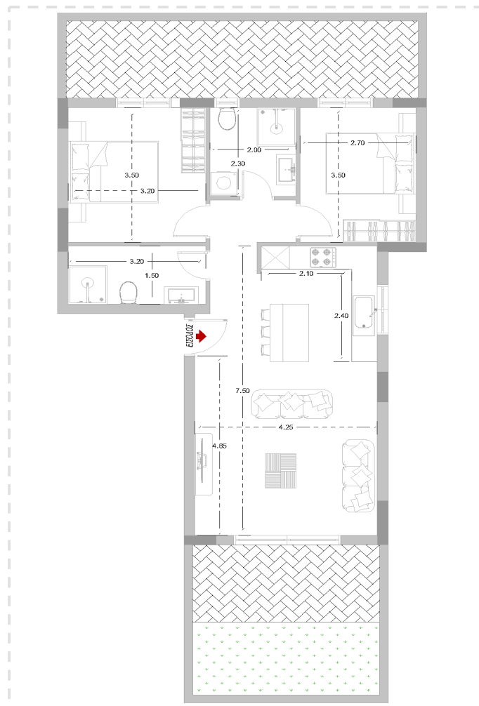
ΚΑΤΟΨΗ ΔΙΑΣΤΑΣΕΙΣ
