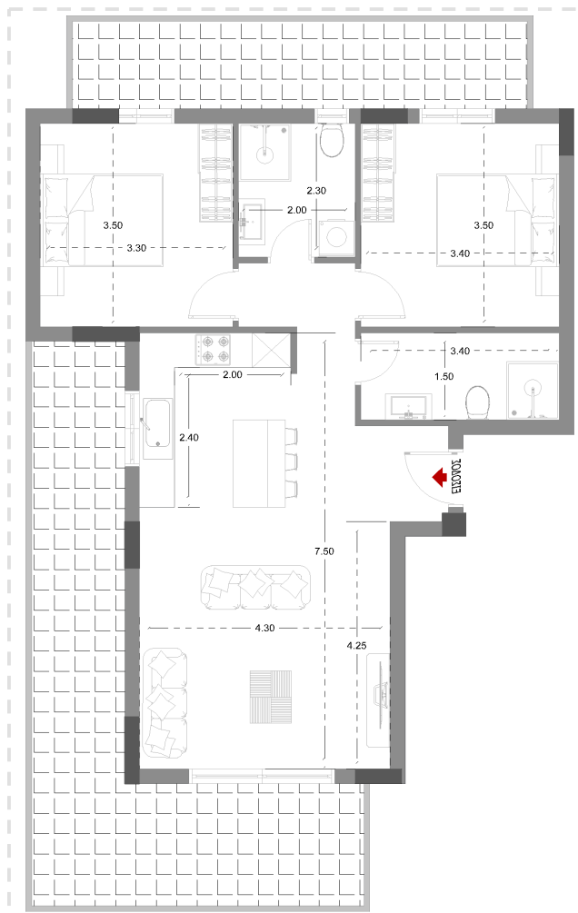
ΚΑΤΟΨΗ ΔΙΑΣΤΑΣΕΙΣ
