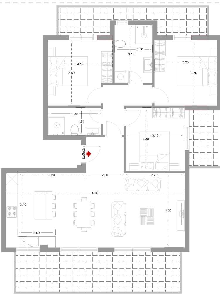
ΚΑΤΟΨΗ ΔΙΑΣΤΑΣΕΙΣ
