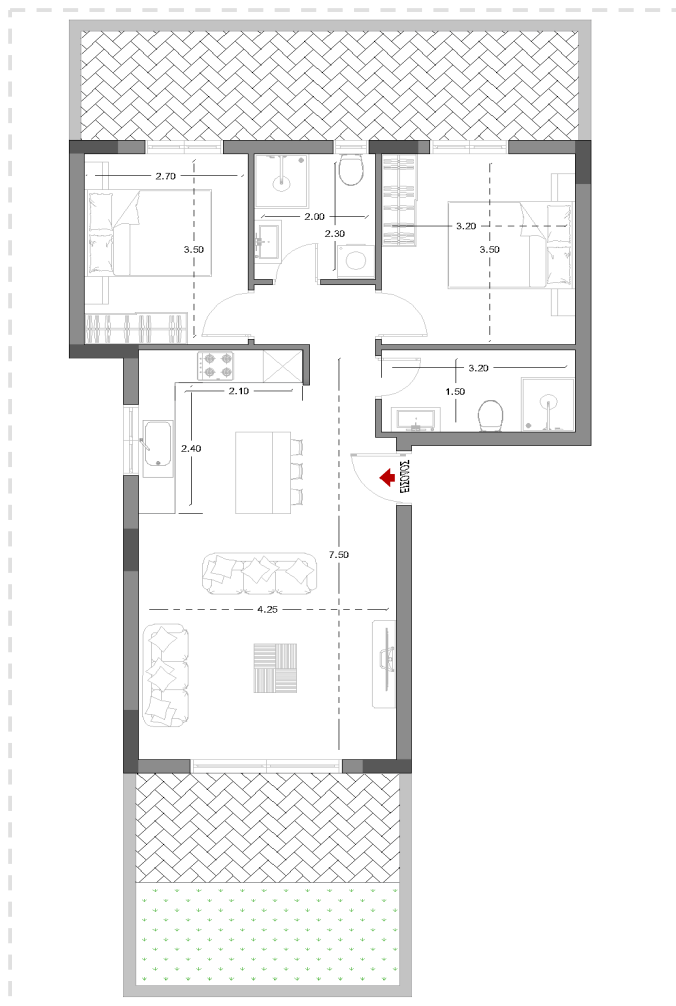
ΚΑΤΟΨΗ ΔΙΑΣΤΑΣΕΙΣ
