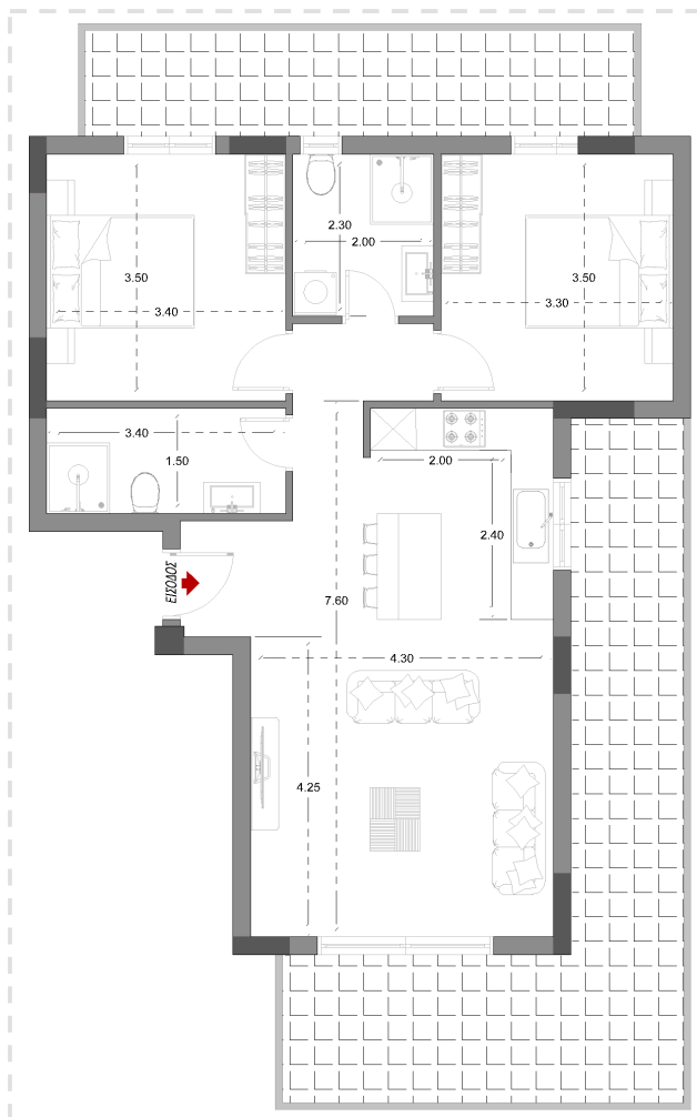
ΚΑΤΟΨΗ ΔΙΑΣΤΑΣΕΙΣ
