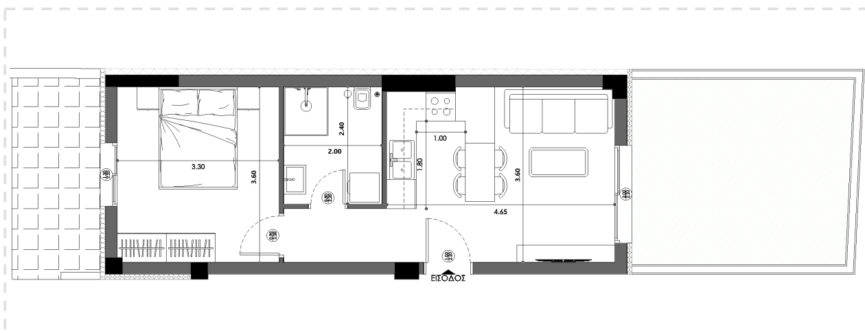
ΚΑΤΩΨΗ ΔΙΑΣΤΑΣΕΙΣ
