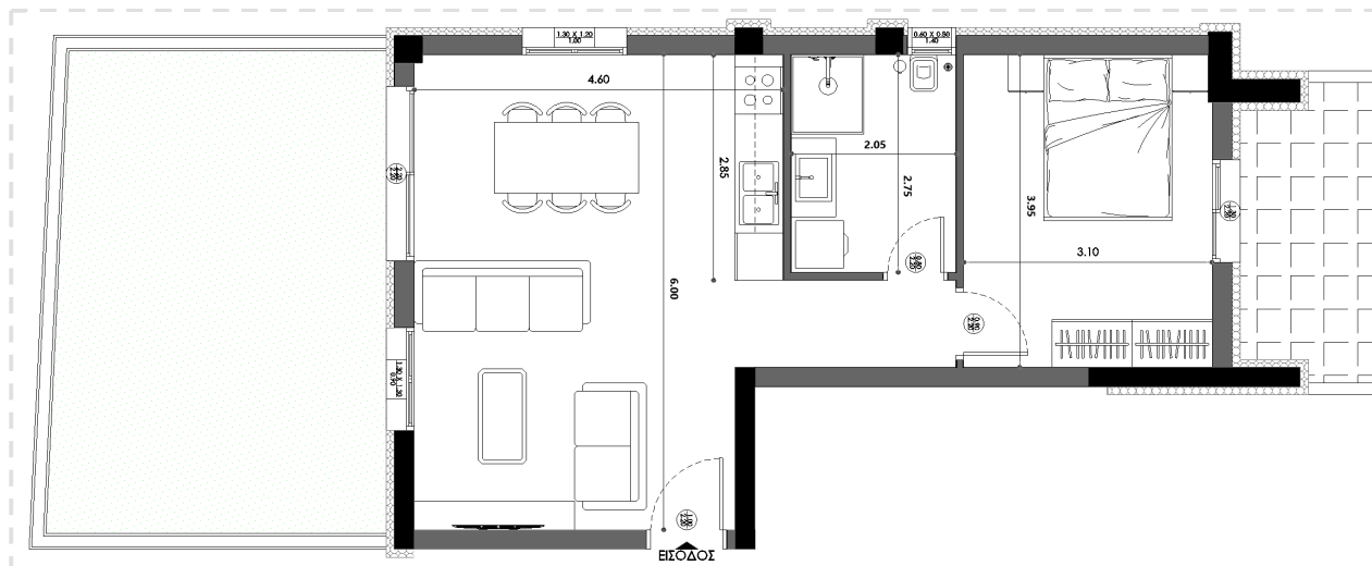
ΚΑΤΟΨΗ ΔΙΑΣΤΑΣΕΙΣ
