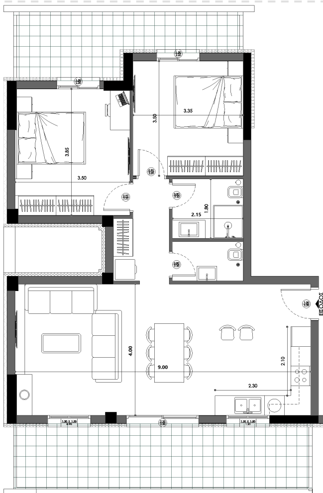
ΚΑΤΟΨΗ ΔΙΑΣΤΑΣΕΙΣ
