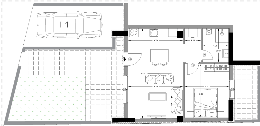
ΚΑΤΟΨΗ ΔΙΑΣΤΑΣΕΙΣ
