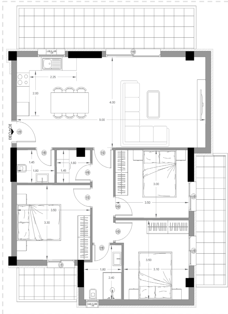
ΚΑΤΟΨΗ — ΔΙΑΣΤΑΣΕΙΣ
