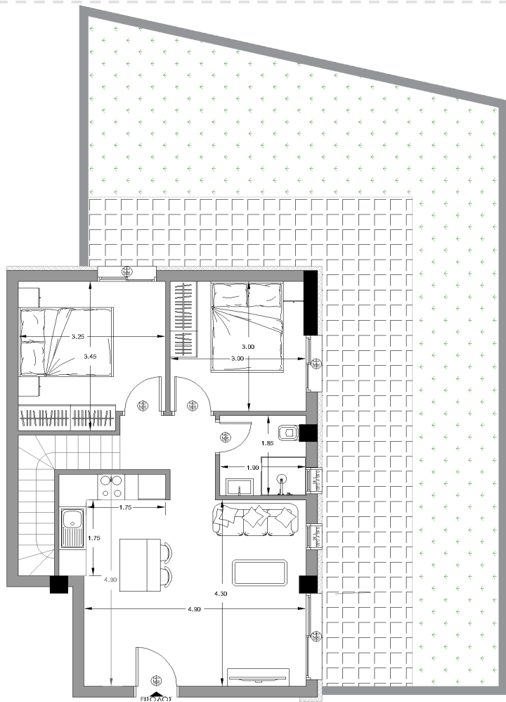
ΚΑΤΟΨΗ — ΔΙΑΣΤΑΣΕΙΣ
