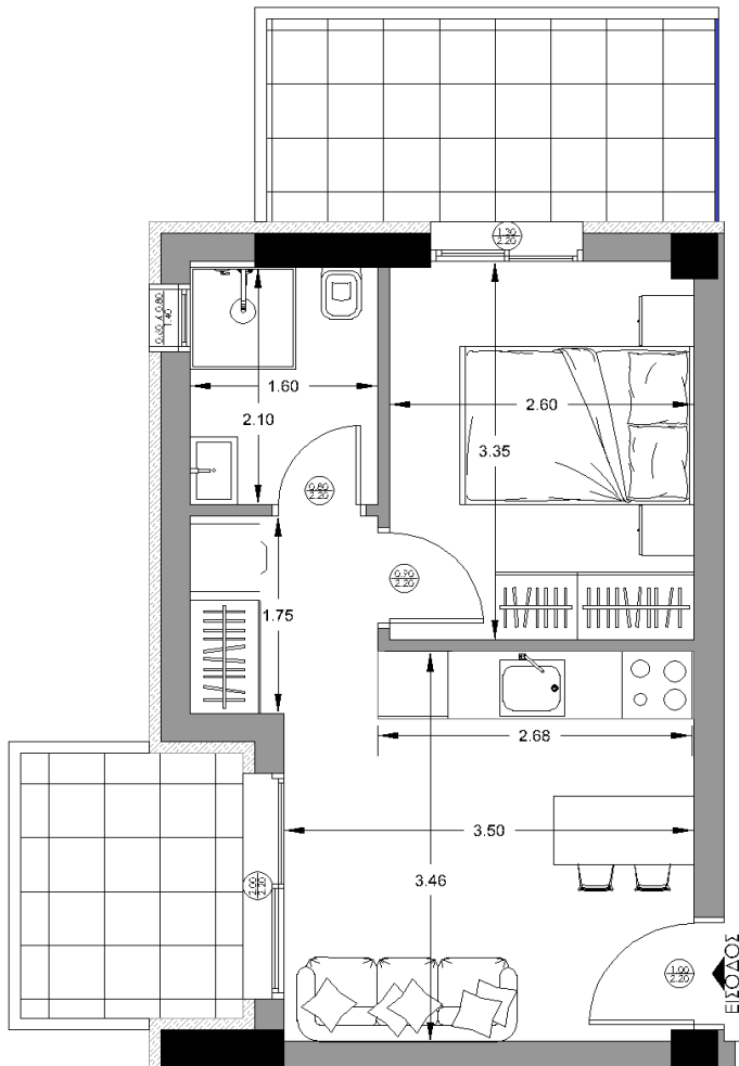
ΚΑΤΟΨΗ — ΔΙΑΣΤΑΣΕΙΣ
