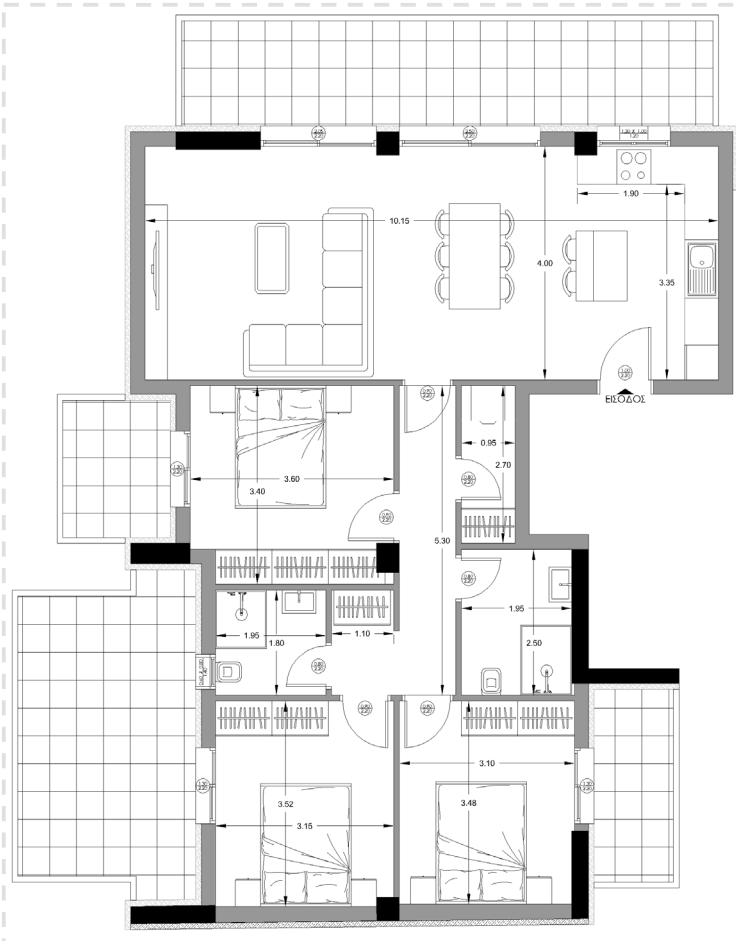
ΚΑΤΟΨΗ — ΔΙΑΣΤΑΣΕΙΣ
