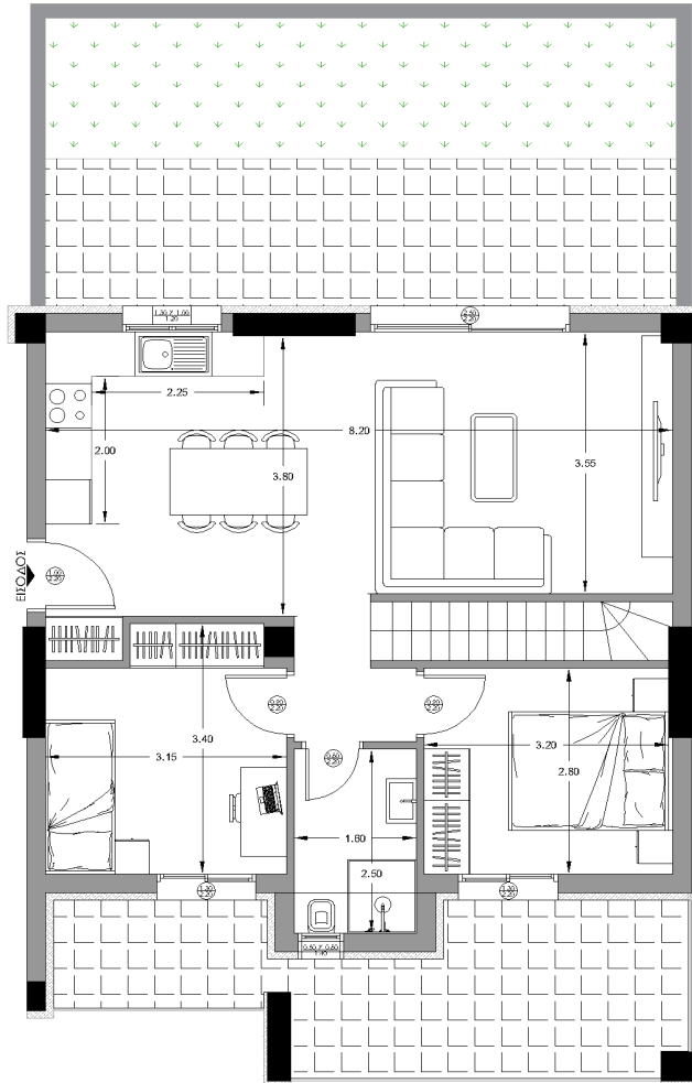
ΚΑΤΟΨΗ — ΔΙΑΣΤΑΣΕΙΣ
