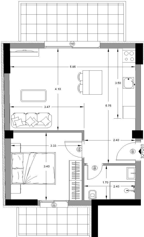
ΚΑΤΟΨΗ — ΔΙΑΣΤΑΣΕΙΣ
