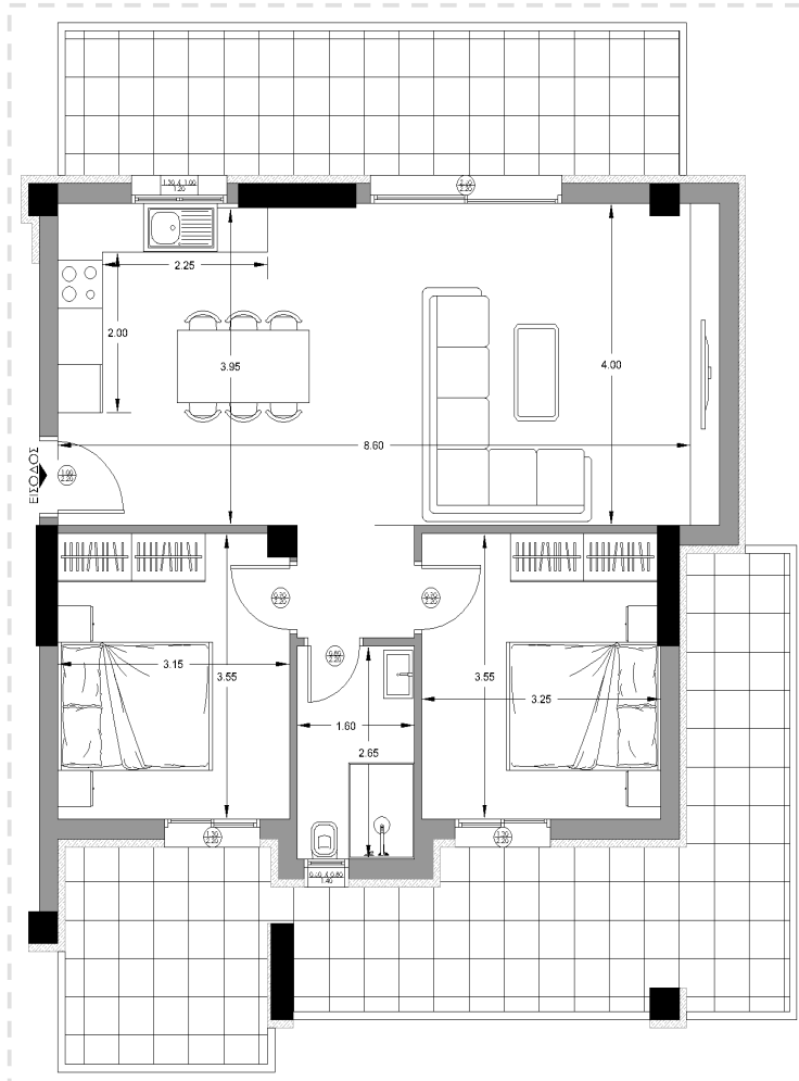
ΚΑΤΟΨΗ — ΔΙΑΣΤΑΣΕΙΣ
