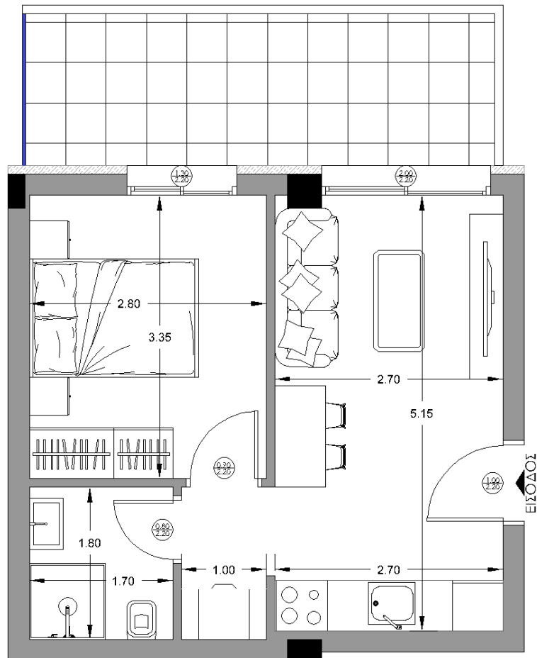
ΚΑΤΟΨΗ — ΔΙΑΣΤΑΣΕΙΣ
