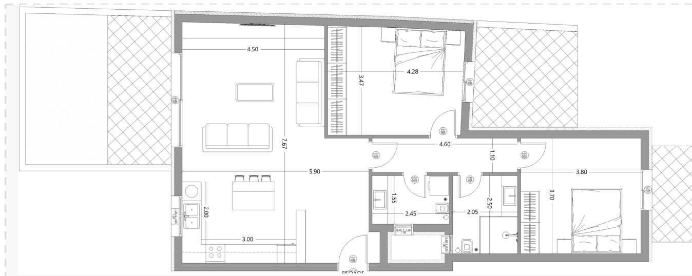
ΚΑΤΟΨΗ ΔΙΑΣΤΑΣΕΙΣ
