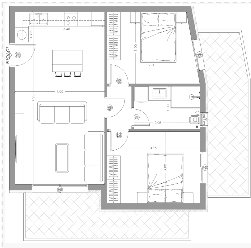
ΚΑΤΟΨΗ — ΔΙΑΣΤΑΣΕΙΣ
