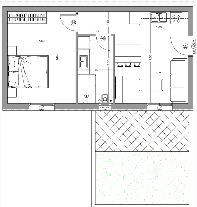
ΚΑΤΟΨΗ — ΔΙΑΣΤΑΣΕΙΣ
