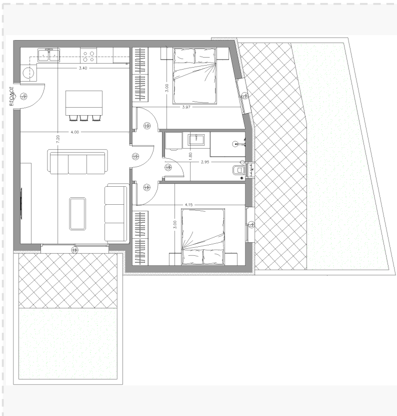
ΚΑΤΟΨΗ — ΔΙΑΣΤΑΣΕΙΣ
