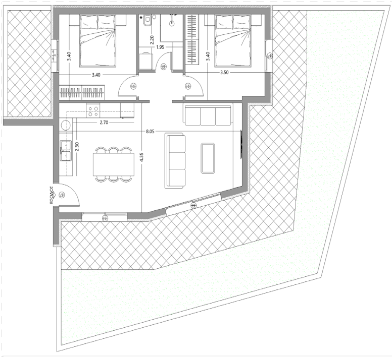
ΚΑΤΟΨΗ — ΔΙΑΣΤΑΣΕΙΣ
