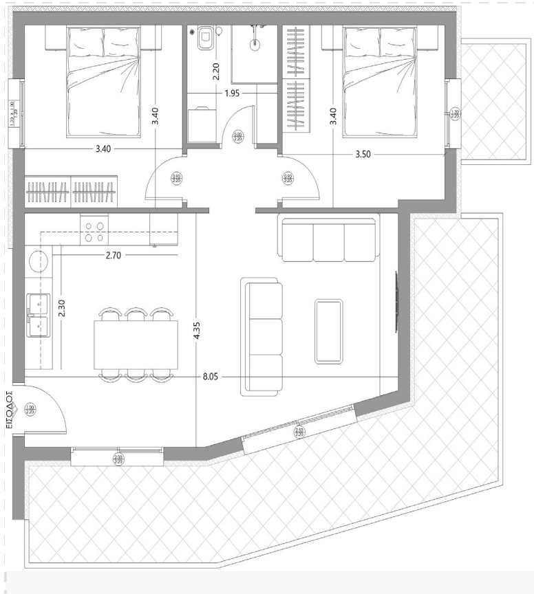
ΚΑΤΟΨΗ — ΔΙΑΣΤΑΣΕΙΣ
