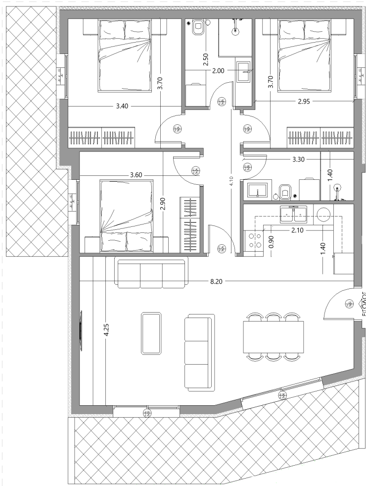
ΚΑΤΟΨΗ — ΔΙΑΣΤΑΣΕΙΣ
