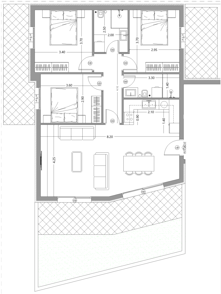
ΚΑΤΟΨΗ — ΔΙΑΣΤΑΣΕΙΣ
